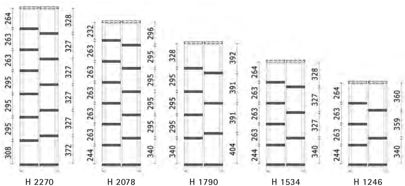
Hauteurs de rayonnages pour les systèmes de rayonnages R.1 à R.4 (y compris vérins de réglage)/exemple de répartition de tablettes = gabarits
